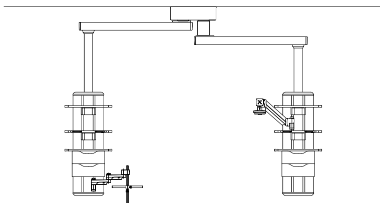
STATIV ZA REANIMACIJU S 2 DVOSTRUKE ZGLOBNE RUKE
